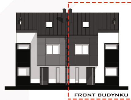
FRONT BUDYNKU
