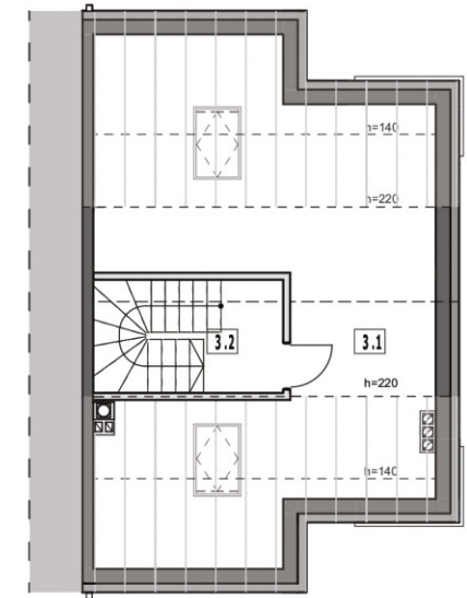
PODDASZE
